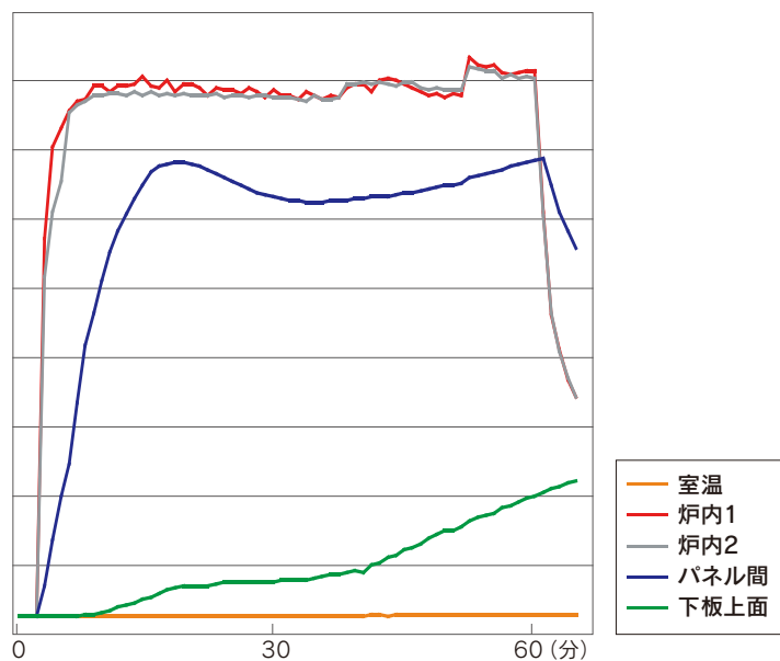
【ケイカル板6mm+FB23mm燃焼試験結果】
