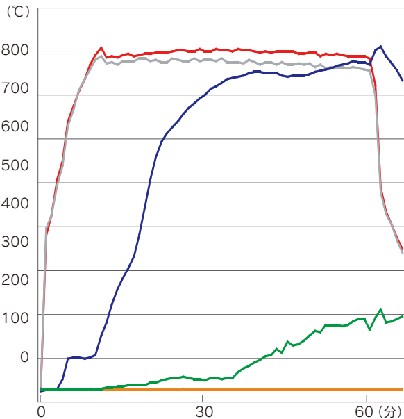
【JFパネル13mm+FB18mm燃焼試験結果】
